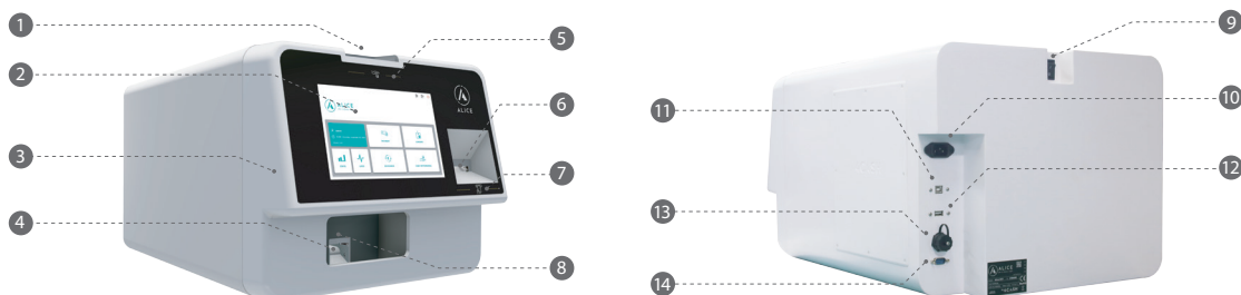
1.Entrada de moedas, 2.Ecrã / touchscreen, 3.Porta da máquina, 4.Saída de moedas, 5.Led indicativo de validador de moedas ativo, 6.Entrada e saída de notas, 7.Led indicativo de validador de notas ativo, 8.Fechadura oculta para abertura da porta, 9. Botão para ligação da máquina [ON/OFF], 10.Conector cabo de alimentação, 11.Conector cabo OTG, 12.Conector cabo USB, 13.Conector Ethernet, 14.Conector de serviço RS232.
